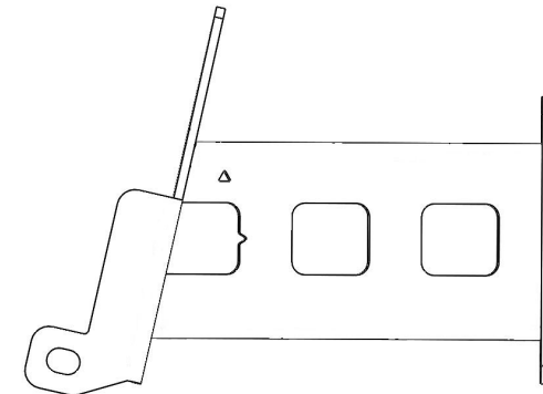
JT SLIDER REAR MOUNT - DS 4JRS2060-06 (x1)
